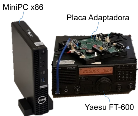
Fig. 1. Plataforma TID-HF com Rádio Yaesu FT-600, expondo placa adaptadora para rádios legados
