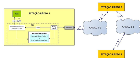
Fig. 6. Setup com três estações rádio usando TID e TDEX
