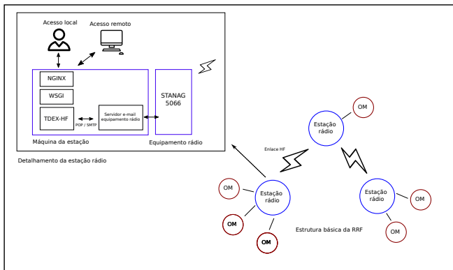
Fig. 5. Arquitetura do TDEX-HF
