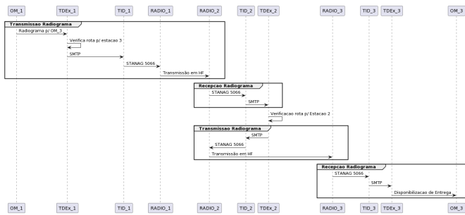
Fig. 7. Diagrama de seqüência da mensagem sendo enviada da estação rádio 1 para estação rádio 3, utilizando TID e TDEX
