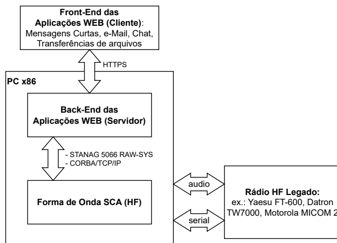
Fig. 2. Sistema de comunicação do TID-HF
