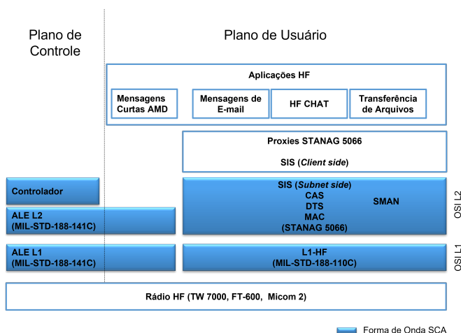
Fig. 3. Arquitetura de referência do TID-HF, destacando a forma de onda SCA e as perspectivas dos planos de controle e de usuário
