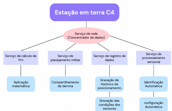
Fig. 5. Estrutura de microsserviços distribuída proposta.
