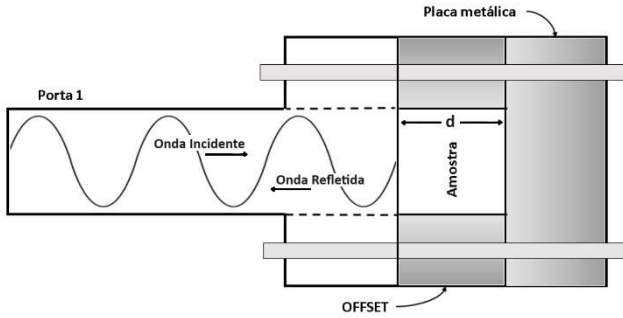
Fig. 3. Representação esquemática da obtenção dos parâmetros utilizados neste trabalho por meio do equipamento VNA. O d representa a espessura da amostra.
