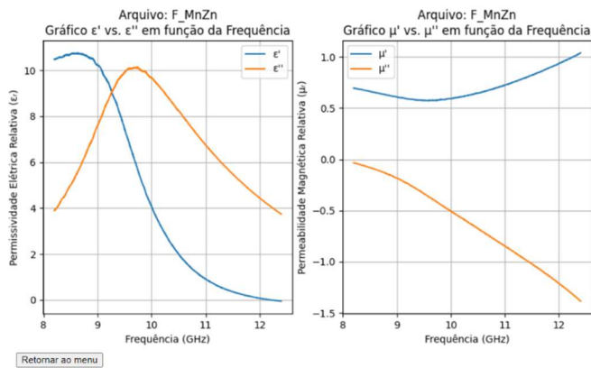
Fig. 7. Tela de plotagem gráfica da permissividade elétrica e permissividade magnética em função da frequência.
