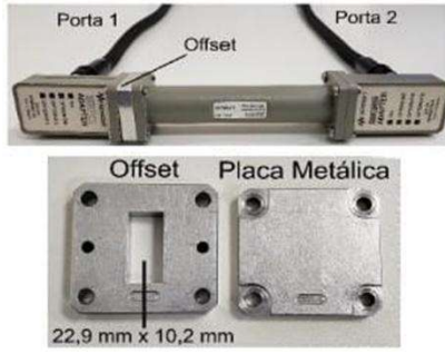
Fig. 2. Foto da vista frontal do porta amostra (Offset) e da placa metálica utilizada para medida no VNA.
