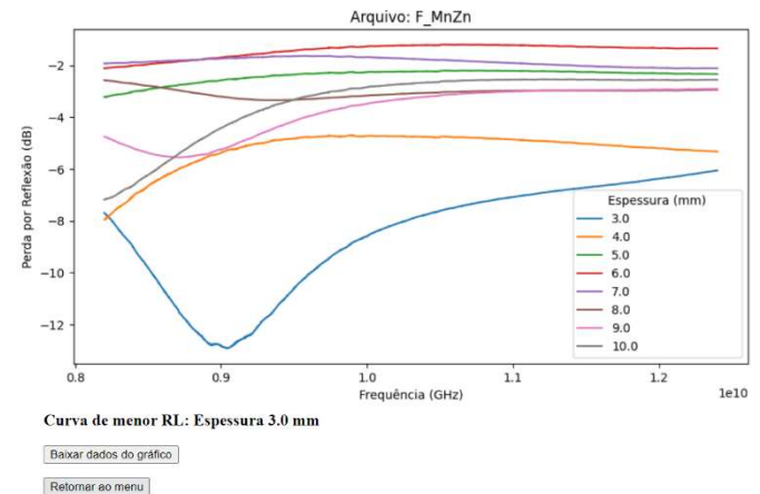
Fig. 9. Tela de plotagem gráfica da perda por reflexão calculada e simulada para diferentes espessuras do material.
